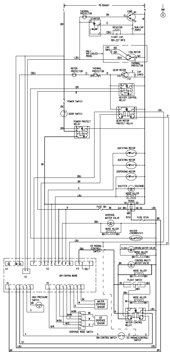
DCM-750BAH-OS, DCM-750BWH-OS
